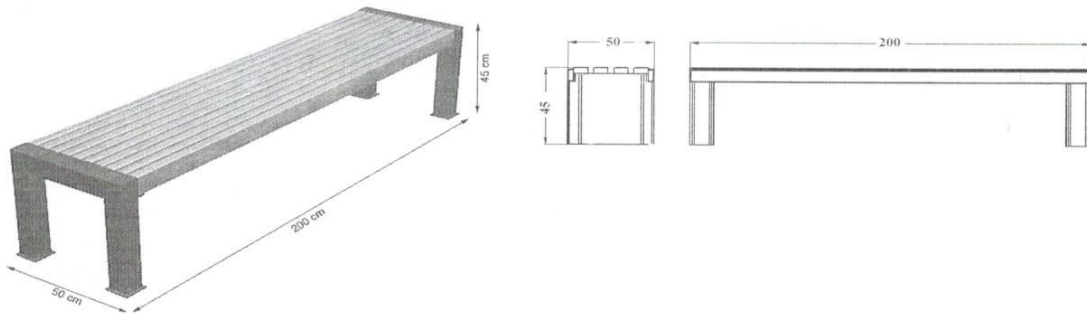
Рис. 1 Парковая скамья переносная деревянная (2 x 0,5 x 0,45)
